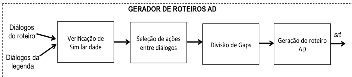
Figura 4: Fluxo do componente gerador de roteiro AD
