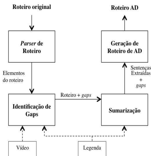
Figura 2: Visão Esquemática do Sistema CineAD
